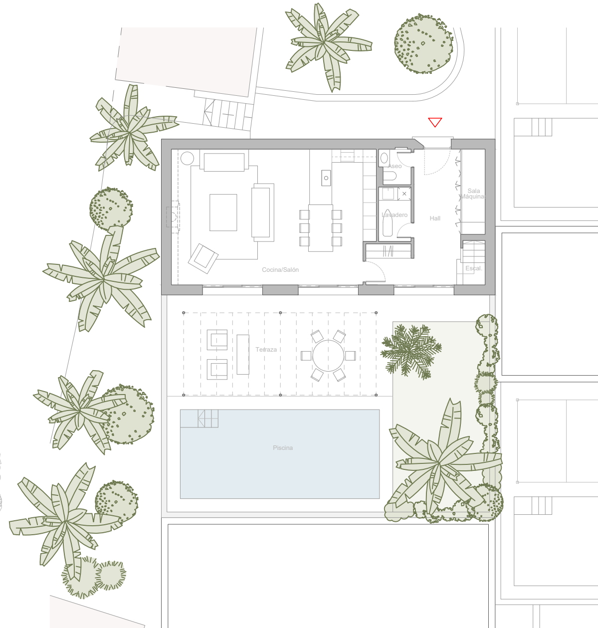
Planta Baja
